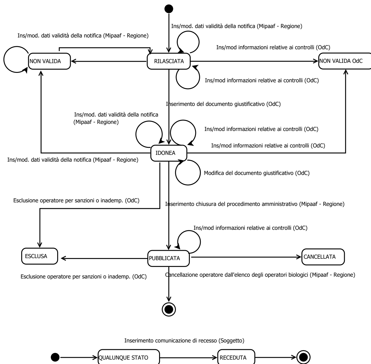
Figura 5 Diagramma di transizione degli stati
